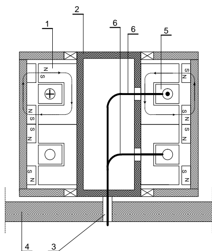
Рисунок 1 – ТВД, поперечний розріз
